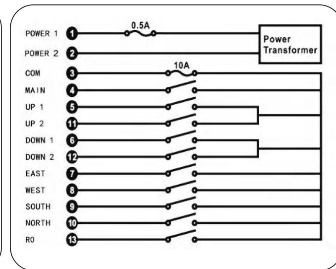
Q602 wiring diagram
