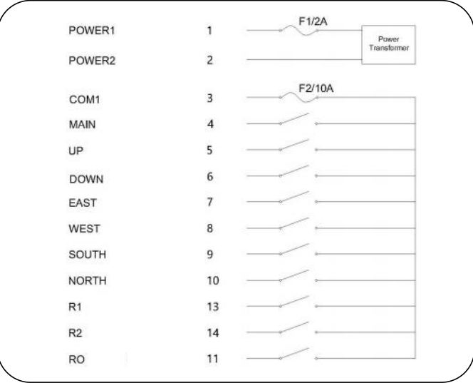
QA600 wiring diagram
